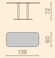
S128-T3M AIDE table
