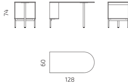
Module L - Table S126-T1
